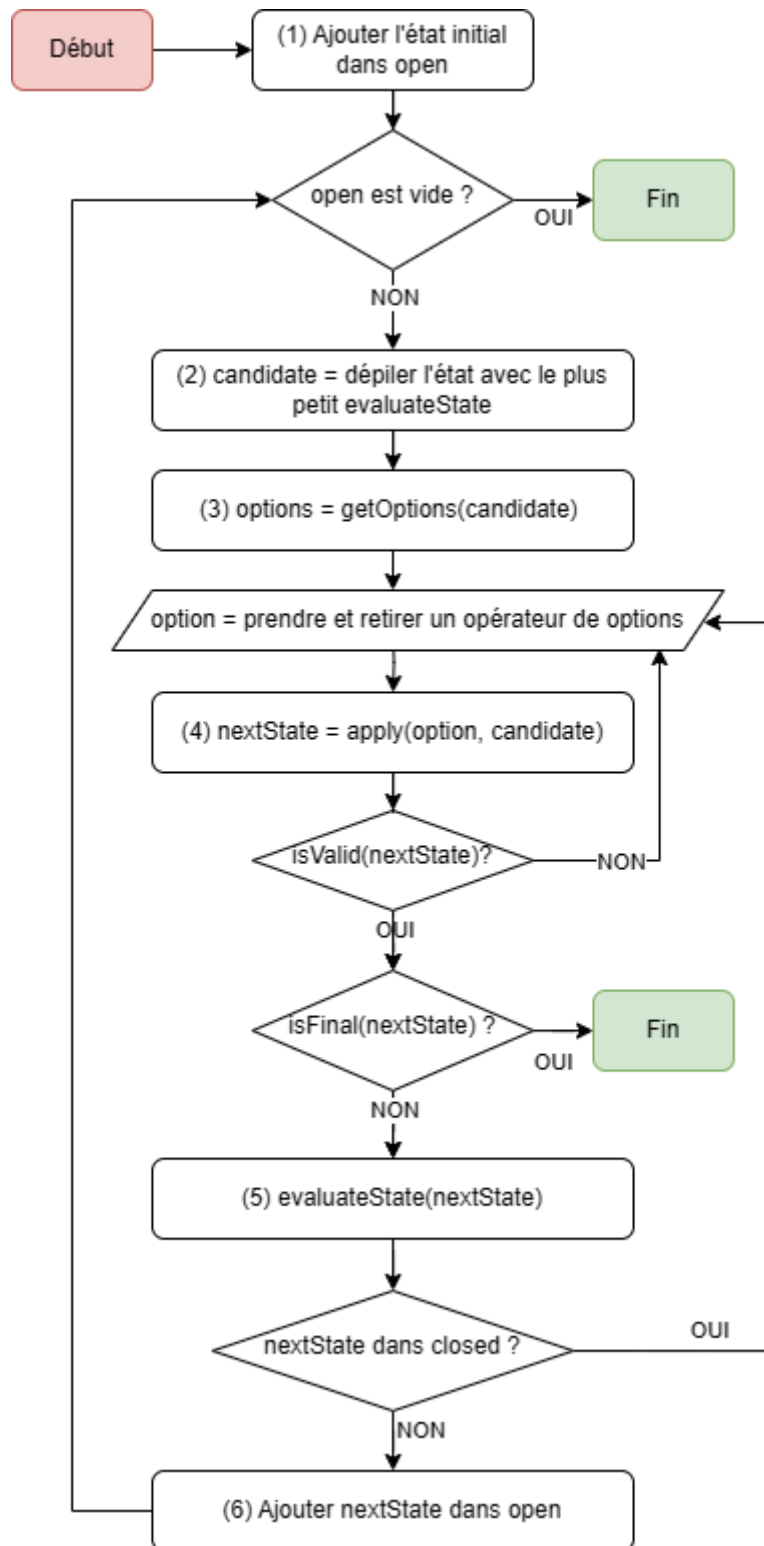
Figure 21: Principe algorithmique d'une recherche dans un espace d'état
