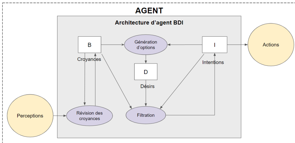
Figure 8 : schéma détaillé de l'architecture BDI
