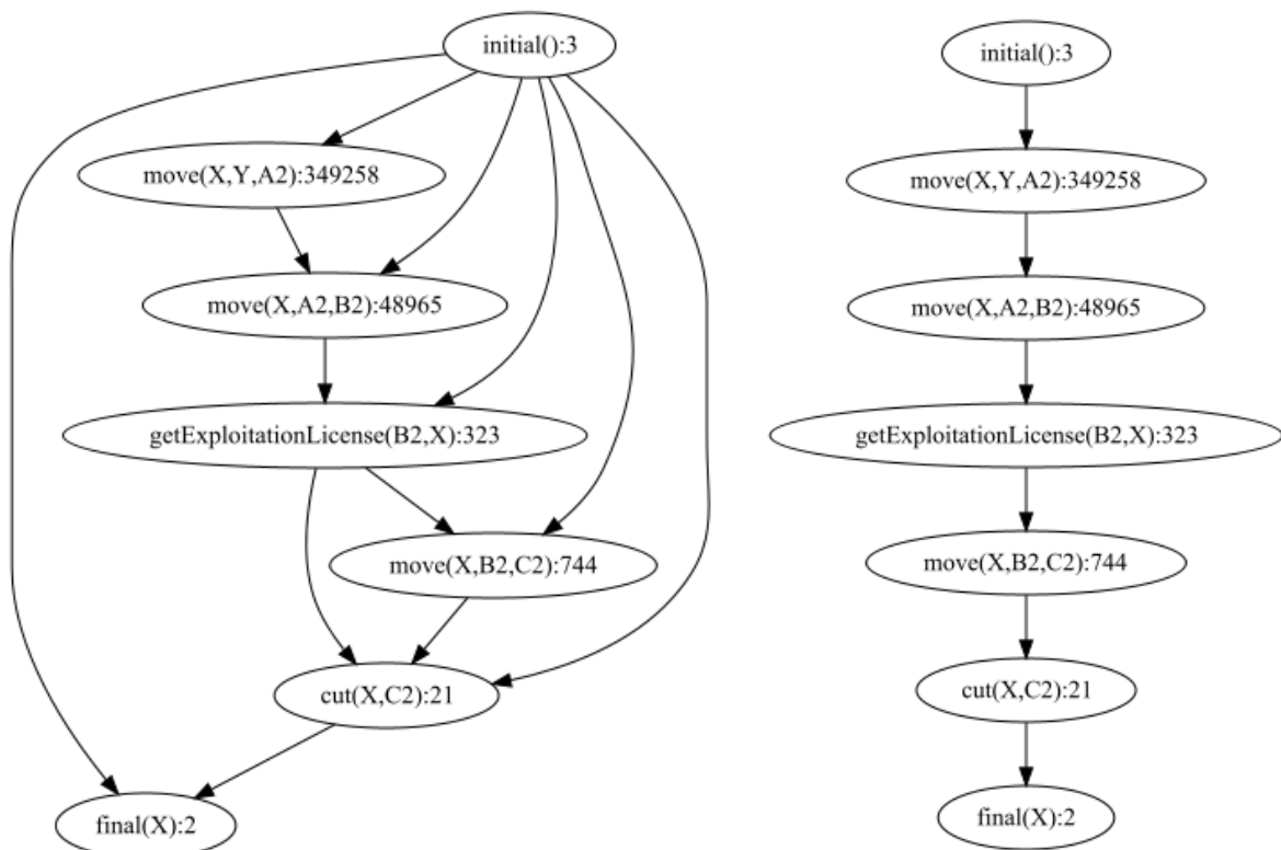
Figure 50: Plan obtenu quand la coupe est permise seulement avec une licence d'exploitation
