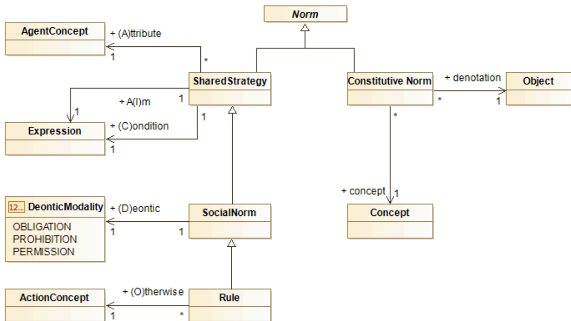
Figure 3: Représentation en diagramme de classe de la grammaire institutionnelle ADICO
