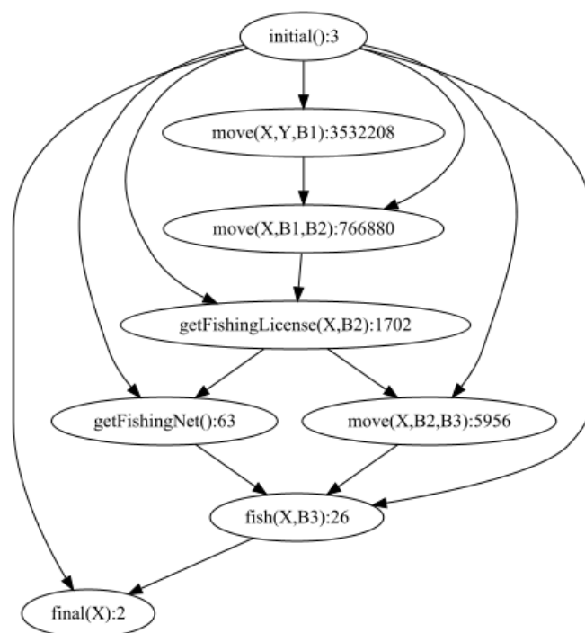
Figure 54: Plan obtenu où si l'agent a une licence, alors il est permis d'avoir un filet de pêche.
