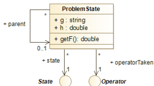
Figure 35: Description du ProblemState qui représente l'arborescence des états dans l'espace de recherche
