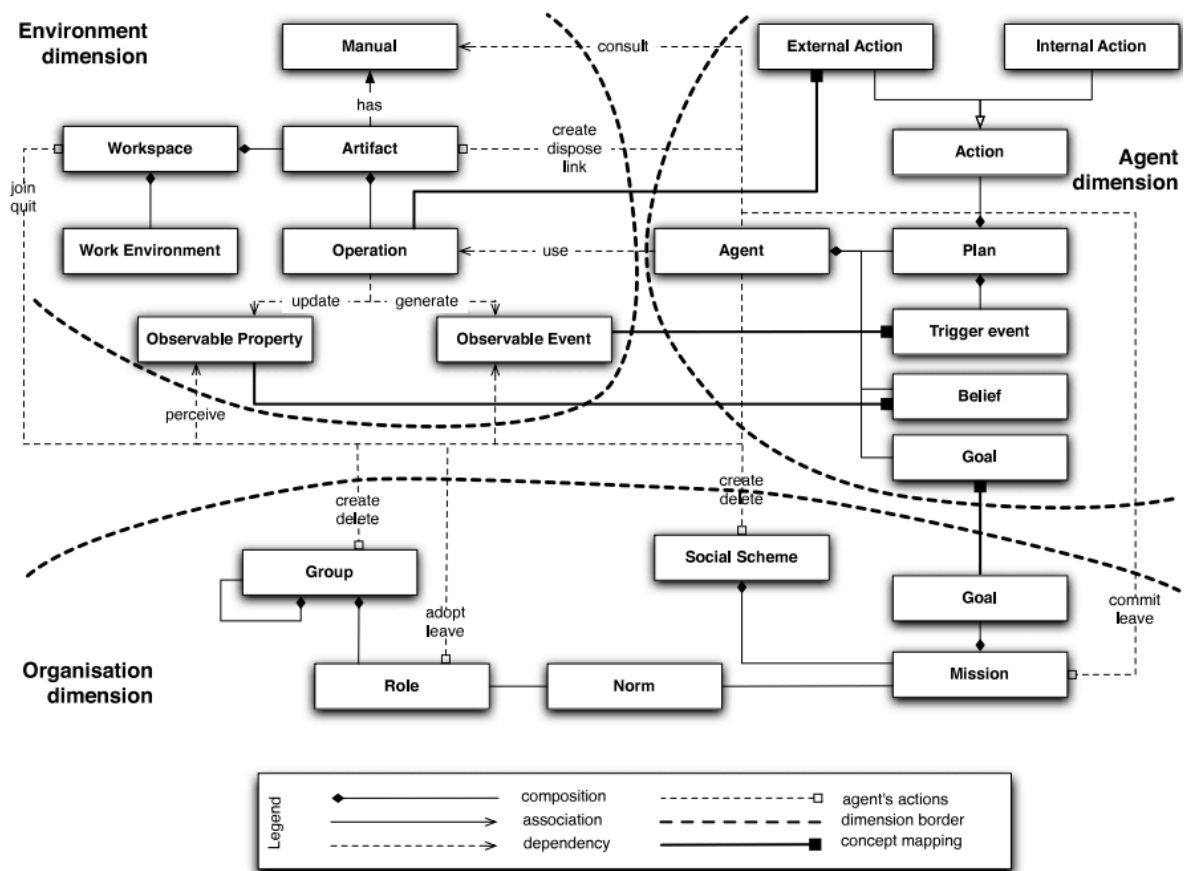
Figure 16: Méta-modèle de JaCaMo et des relations et correspondances entre les concepts des différentes dimensions, présenté dans [Boissier et al., 2013]
