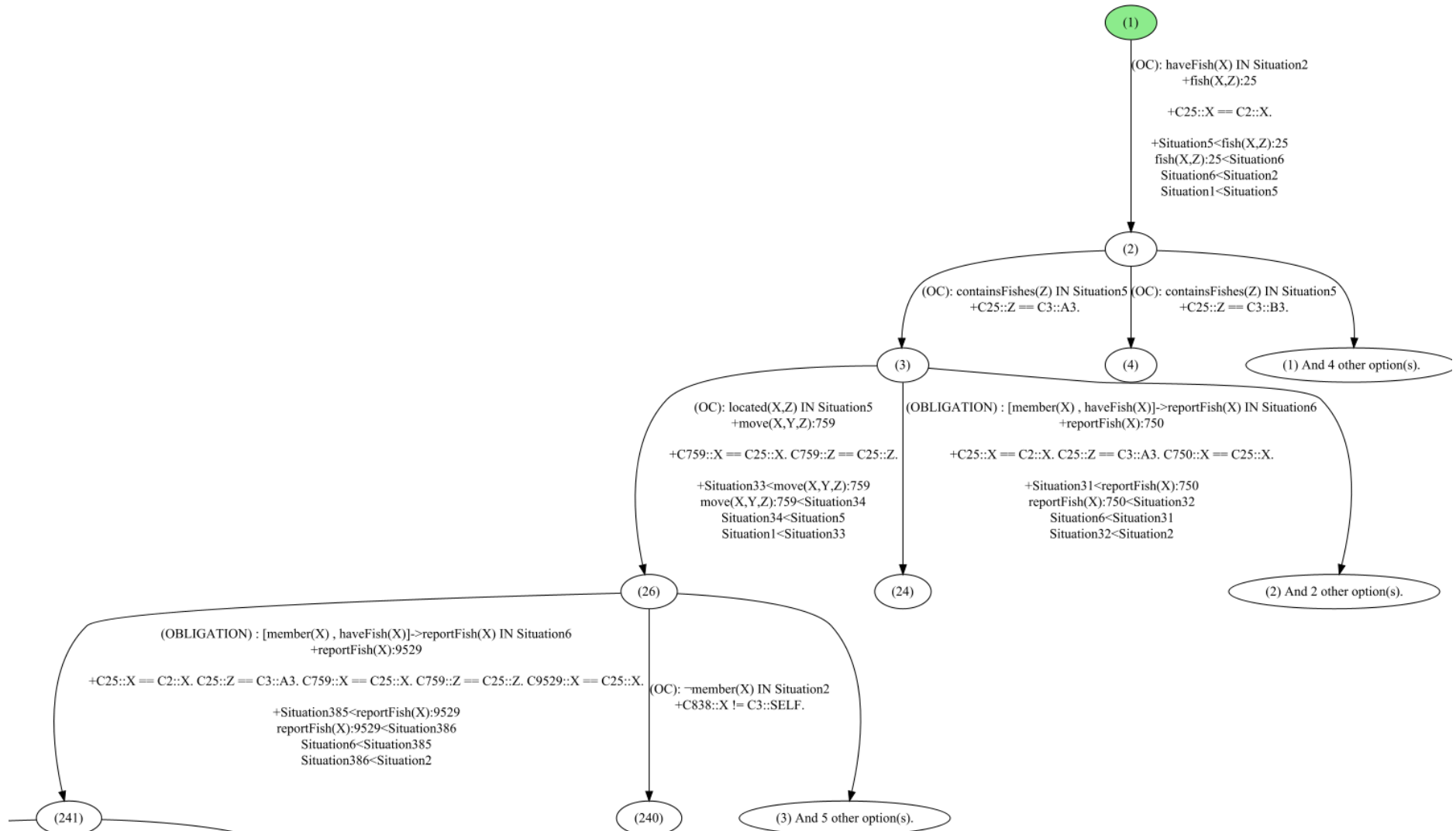
Annexe 3 : Parcours de l'espace de recherche quand on a l'obligation de déclarer ses prises quand l'agent a fini de pêcher
