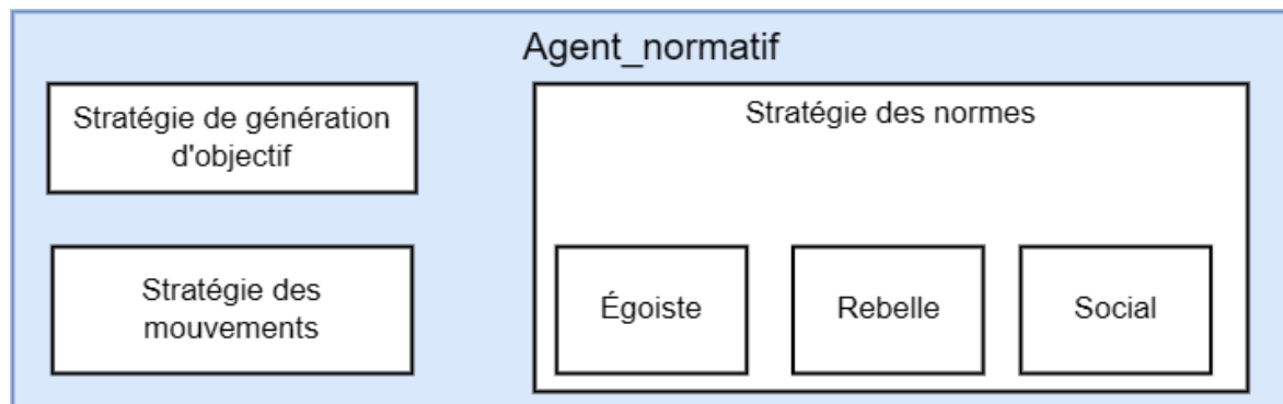
Figure 17: Structures à définir pour créer un agent normatif dans JSAN
