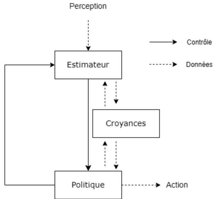
Figure 23: Cycle de perception-action d'un agent POMDP, adapté de [Schut et al., 2012].
