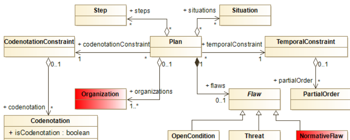
Figure 34: Nos extensions sur l'état classique du POP (en rouge)
