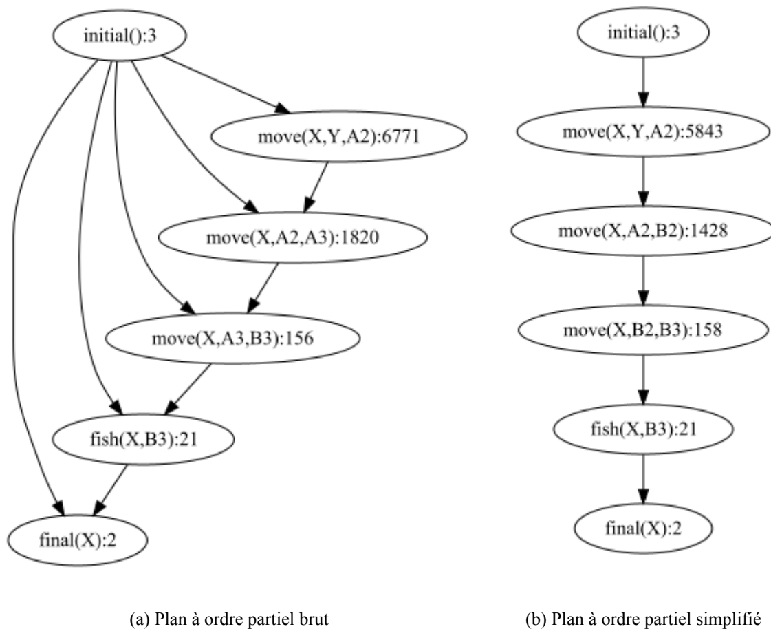
Figure 44: Comparaison des comportements obtenus avec et sans interdiction sur la pêche
