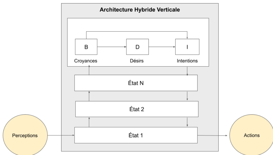
Figure 11 : Illustration de l'architecture hybride verticale
