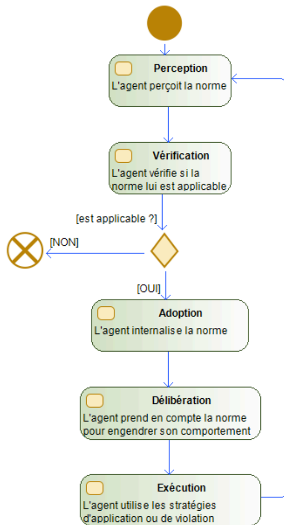
Figure 12: Cycle de vie des normes dans les architectures d'agent normatives, adapté de [Mahmoud et al., 2014]
