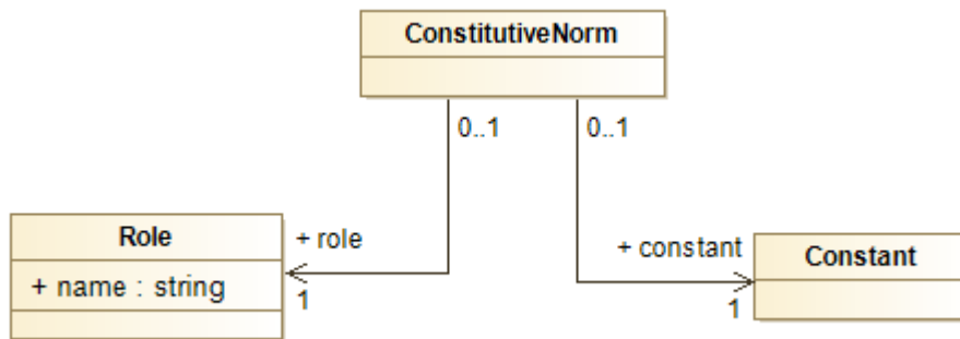
Figure 31: Syntaxe abstraite d’une norme constitutive
