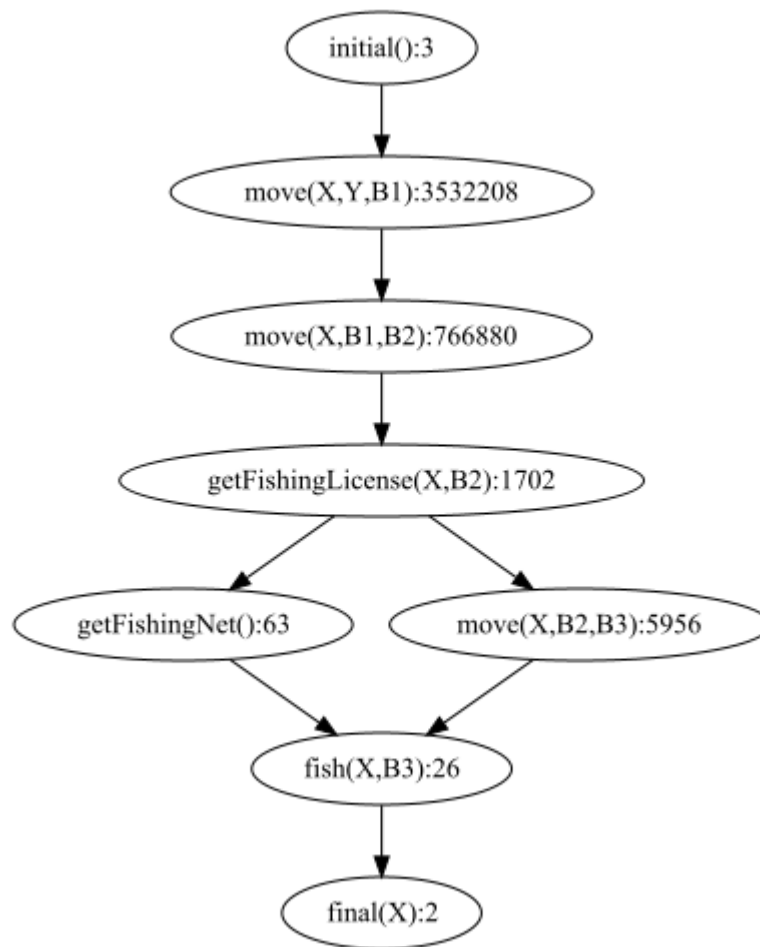
Figure 55: Plan simplifié obtenu avec la permission : si on a une licence de pêche, alors il est permis d’avoir un filet de pêche.
