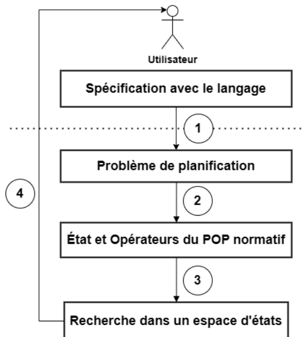
Figure 25: Les différentes étapes de traduction de la spécification du problème de planification à l'obtention du plan
