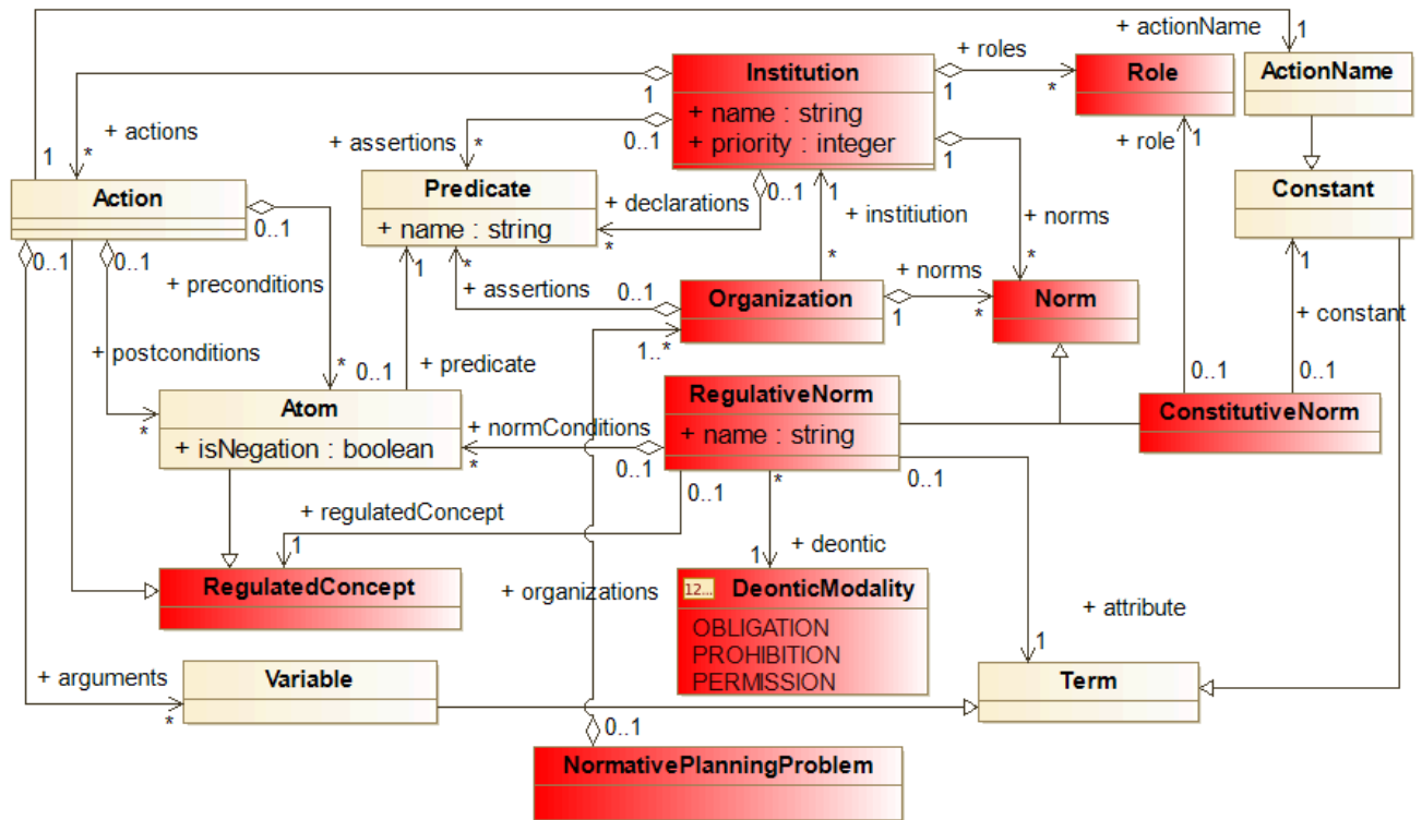
Figure 28: Syntaxe abstraite d'un problème de planification normatif avec nos contributions (en rouge)
