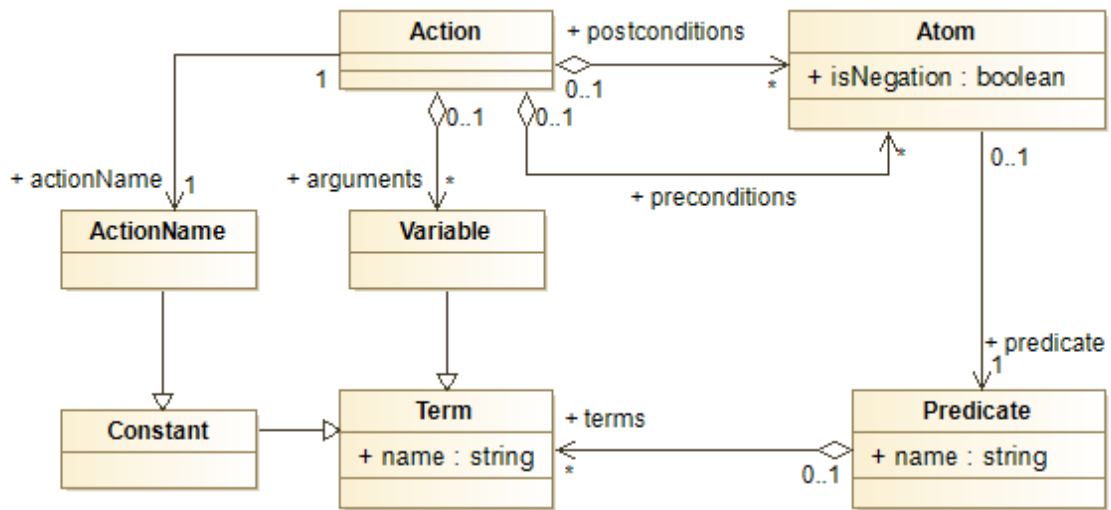
Figure 29: Syntaxe abstraite d'une action dans le présent travail.
