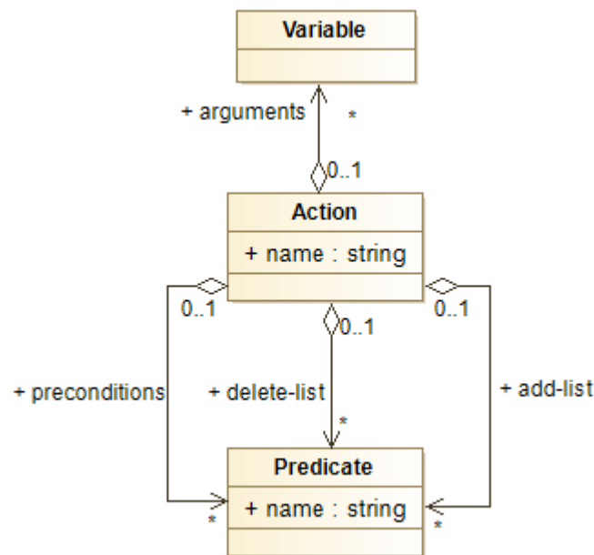
Figure 19: Structure d'une action STRIPS classique
