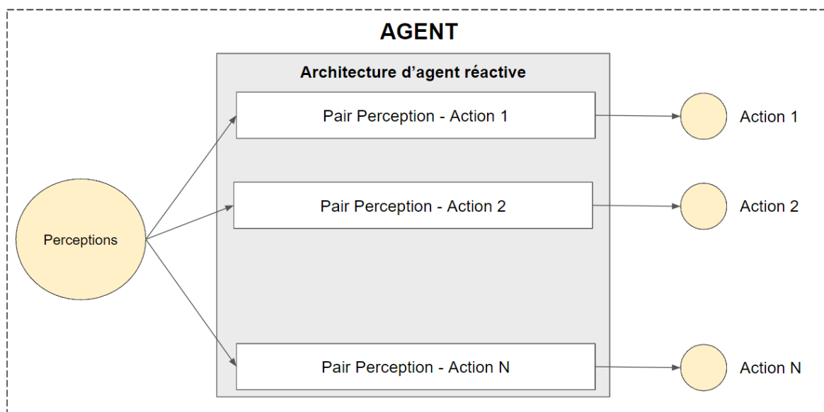
Figure 9: Représentation de l'architecture réactive
