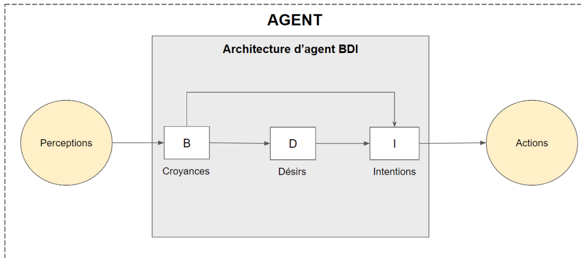
Figure 7: Structure globale des composants de l'architecture BDI
