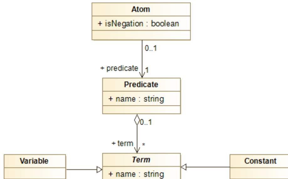
Figure 26 : Syntaxe abstraite des atomes et des prédicats
