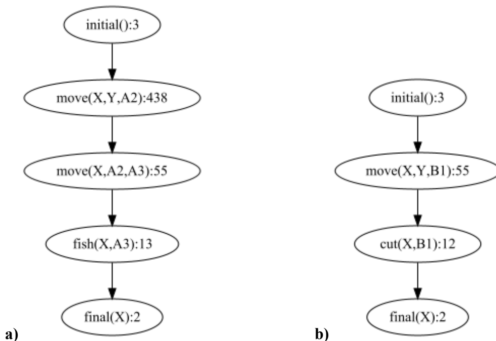
Figure 39: Plans obtenus, sans objectifs et avec uniquement l'obligation : a) d'avoir du poisson, et b) d'avoir du bois
