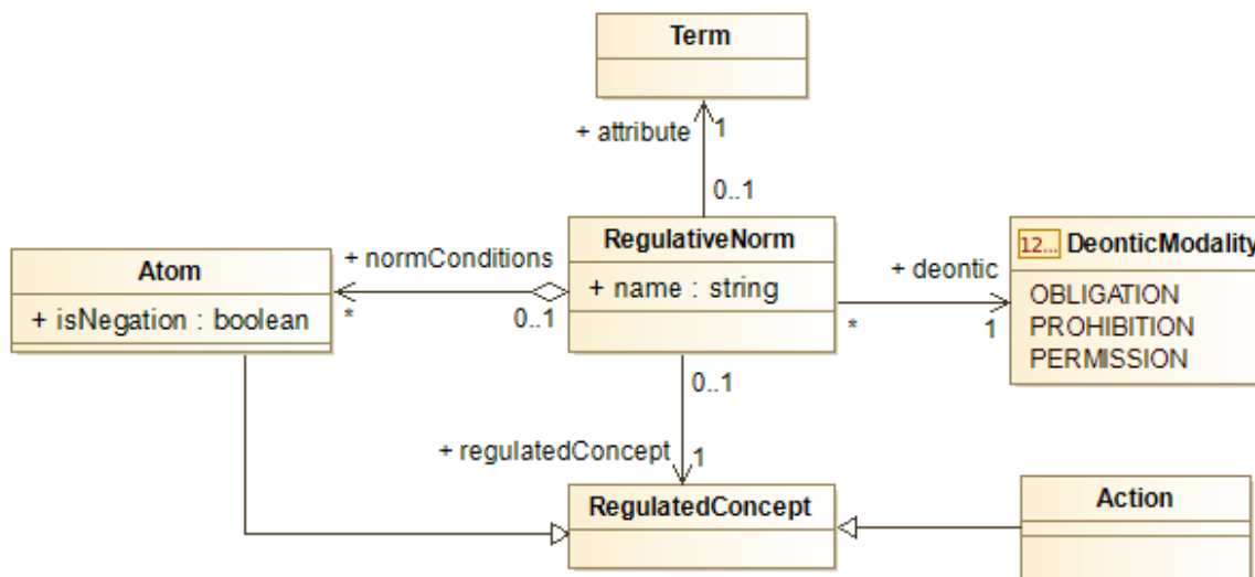
Figure 30: Syntaxe abstraite d’une norme régulatrice
