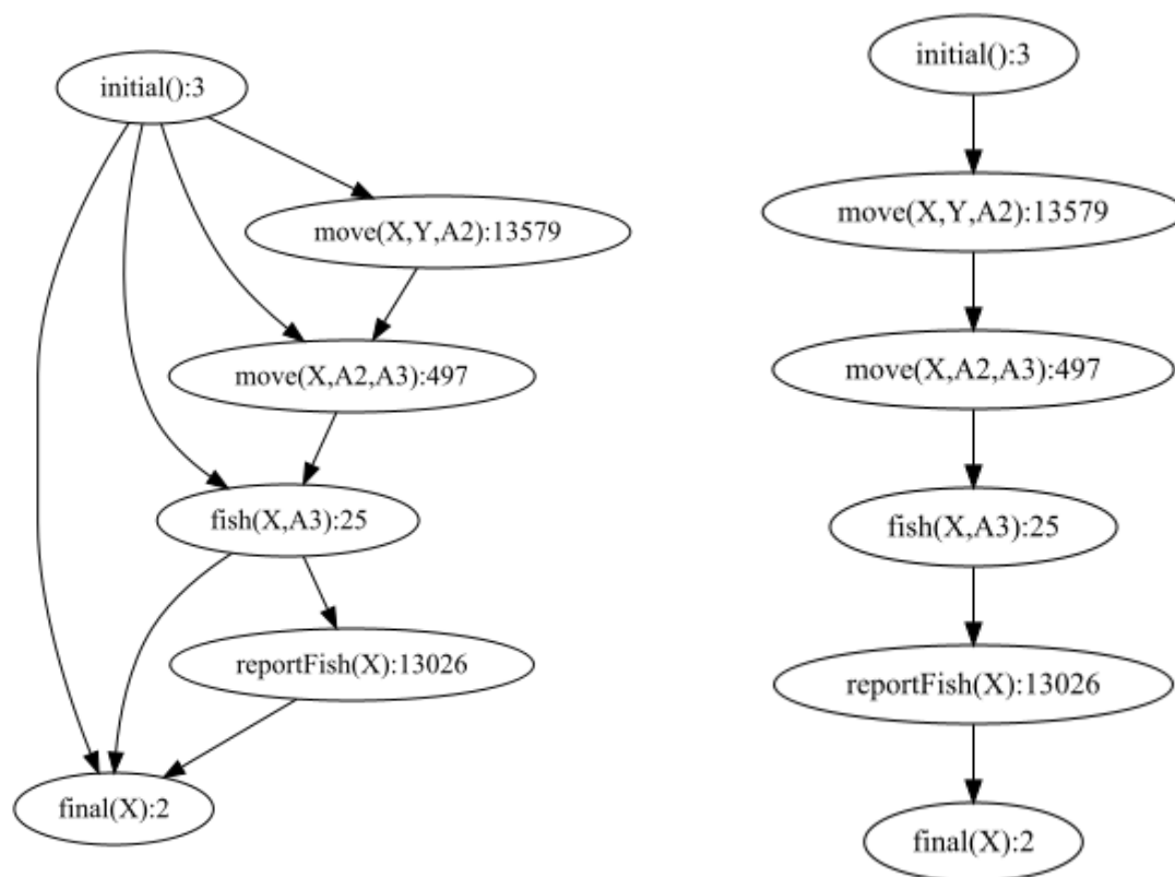
Figure 41 : Représentation simplifiée du plan obtenu avec l'obligation de trouver du poisson et de déclarer ses prises avec l'action reportFish .
