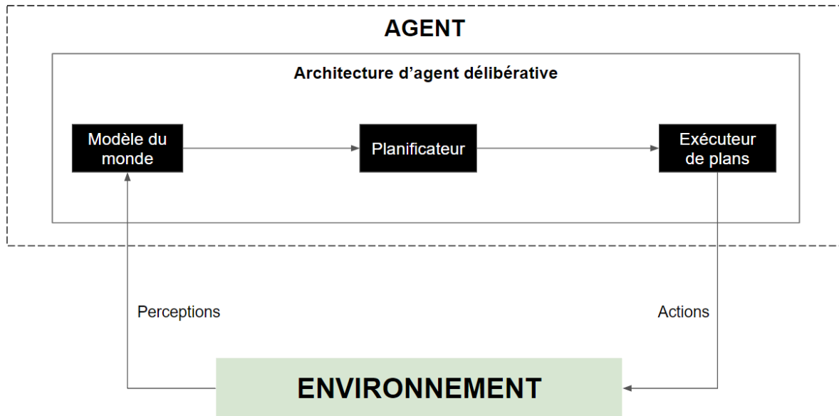
Figure 6: Schéma des composants d'une architecture délibérative [Uliuru, 2011]
