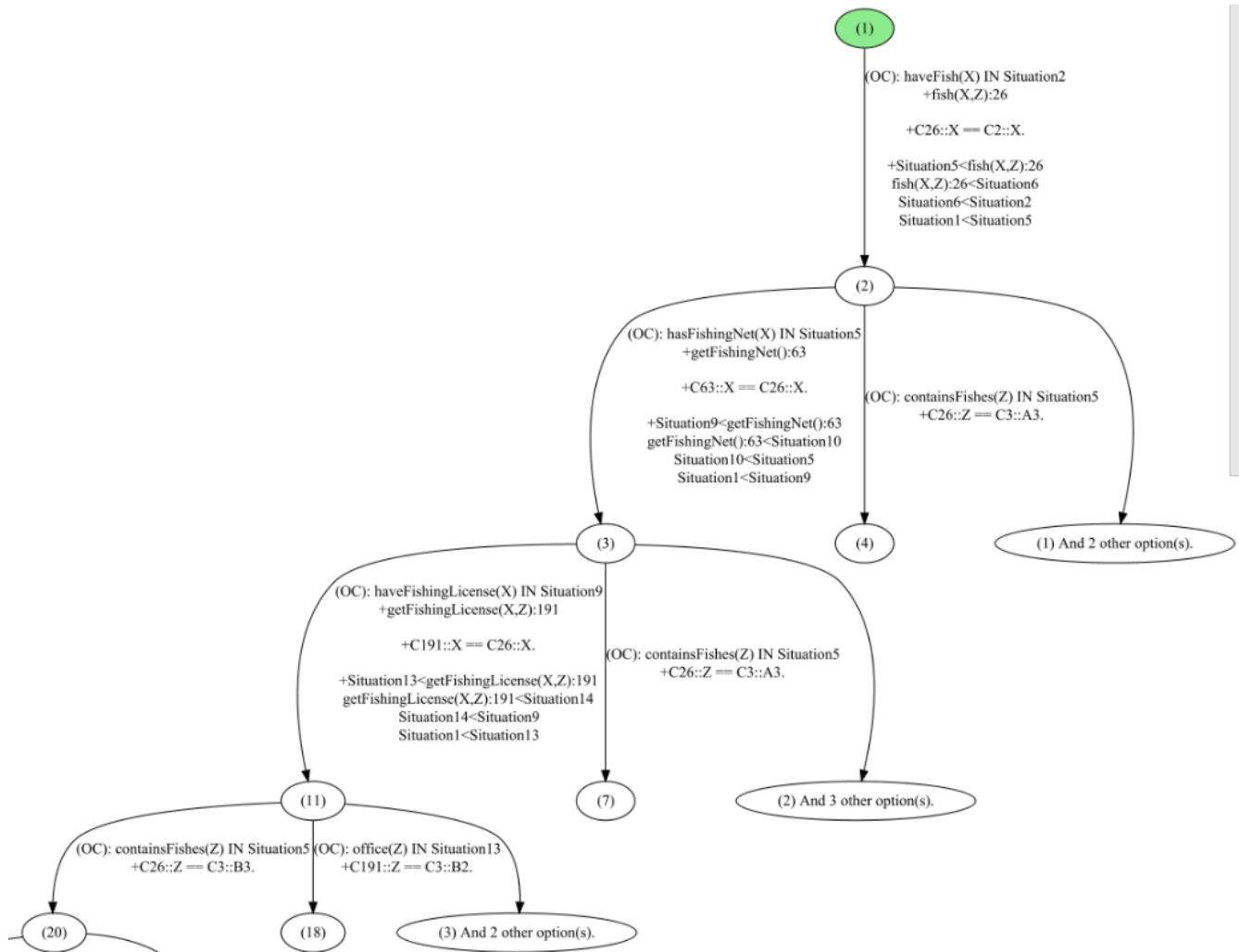
Annexe 1 : Aperçu d'une portion de l'espace de recherche quand la pêche requiert un filet de pêche, mais que ce filet est seulement permis quand on a une licence.
