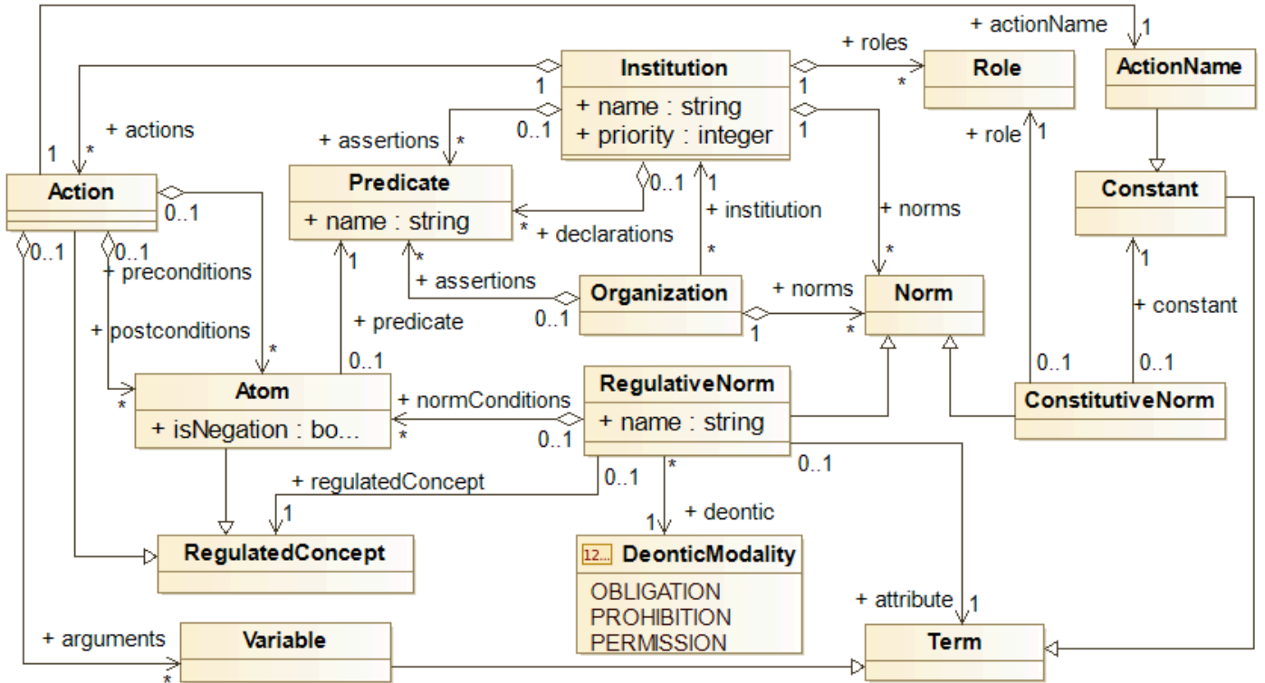
Figure 33: Syntaxe abstraite complète des organisations et des institutions
