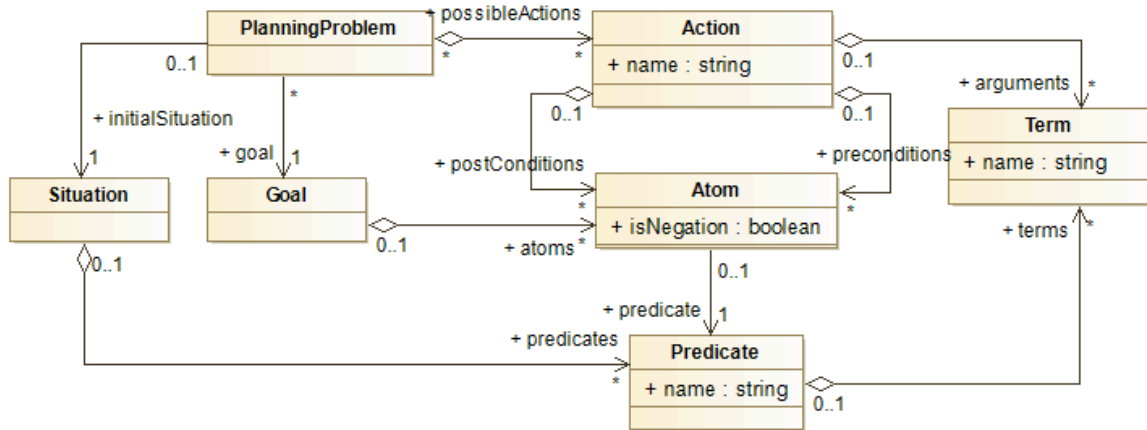
Figure 27: Syntaxe abstraite d’un problème de planification classique
